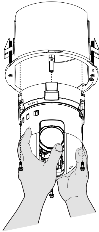
Figura 9. Instalación del accionamiento de domo: modelos empotrados en techo
