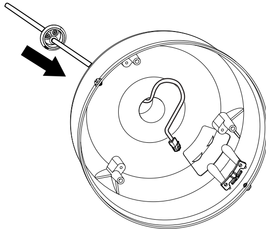
Figura 10. Accionamiento de domo con ojal instalado en la parte posterior
