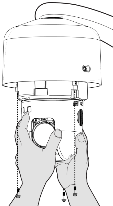
Abbildung 12. Installation des Dome-Antriebs: Modelle zur Hängemontage
